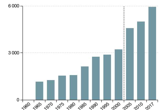
Graphique 59 : évolution de la consommation d'électricité des secteurs résidentiel et tertiaire dans le Massif central, par habitant
