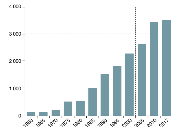
Graphique 81 : évolution de la puissance électrique installée des remontées mécaniques des communes supports de stations de ski du Jura
