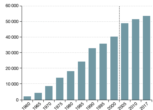
Graphique 38 : évolution de la consommation d'électricité des secteurs résidentiel et tertiaire dans les Pyrénées, par habitant
