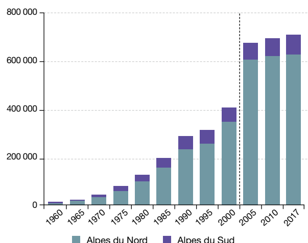
Graphique 18 : évolution de la puissance électrique installée des remontées mécaniques des communes supports de stations de ski des Alpes
