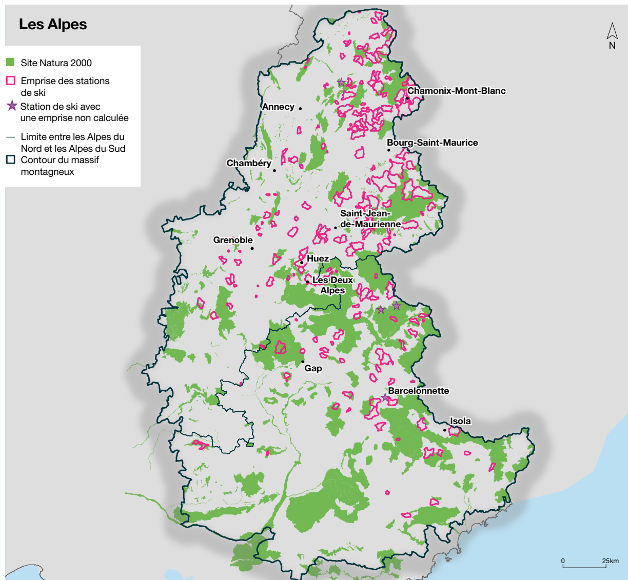
Carte 11 : interactions entre stations de ski et aires protégées (sites Natura 2000) dans les Alpes, en 2017
