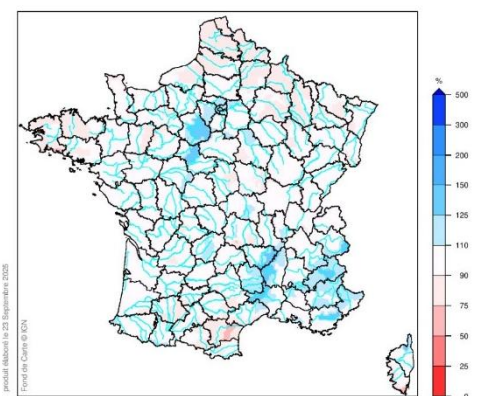
Rapport à la normale du cumul de précipitations sur l'année hydrologique 2024 – 2025
