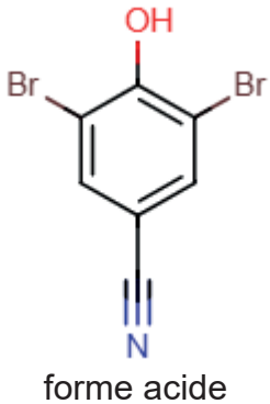
bromoxynil
